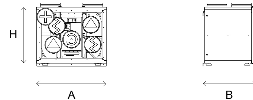
WIDOK OD STRONY OBSŁUGOWEJ VIEW FROM THE OPERATING SITE
