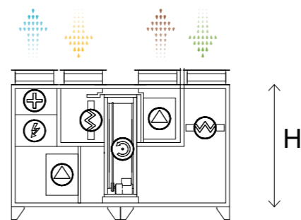
WIDOK OD STRONY OBSŁUGOWEJ WERSJA LEWA
