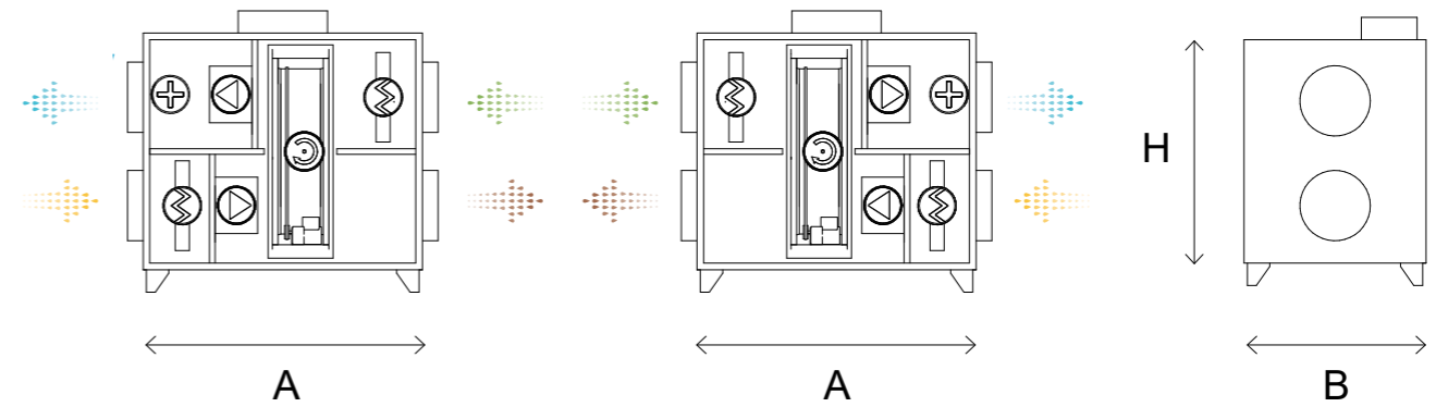
WIDOK OD STRONY OBSŁUGOWEJ WERSJA LEWA
