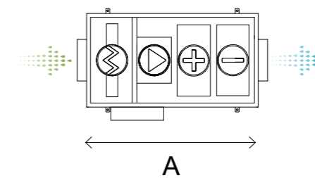
WIDOK Z GÓRY (przeciwny do strony obsługowej) WERSJA PRAWA TOP VIEW (opposite to the operating site) RIGHT VERSION
