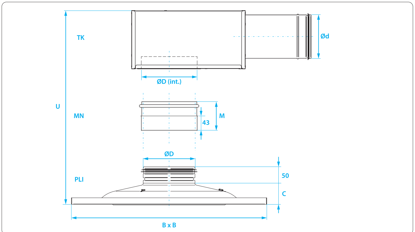
Figure 06 - Dimensions PLI + TK 1-2-step + MN
