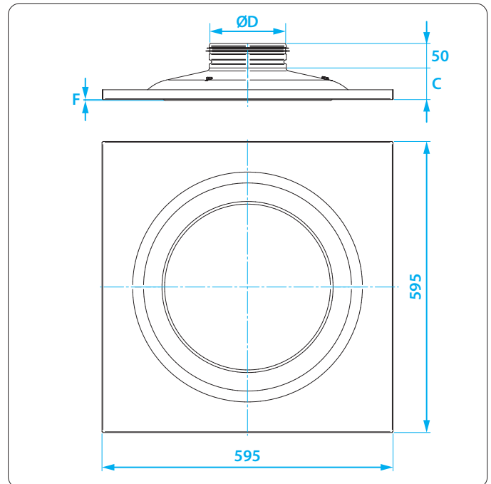
Figure 02 - Dimensions PLI
