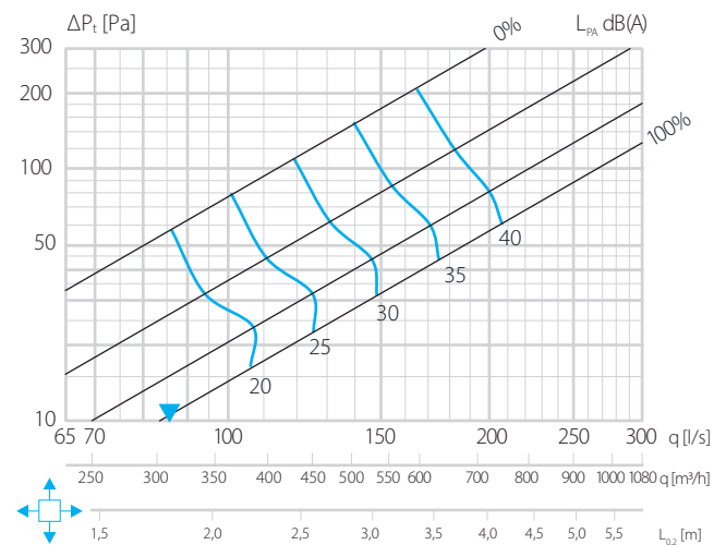
Diagram 03 - PLI-250 - TK-250-250 sound
