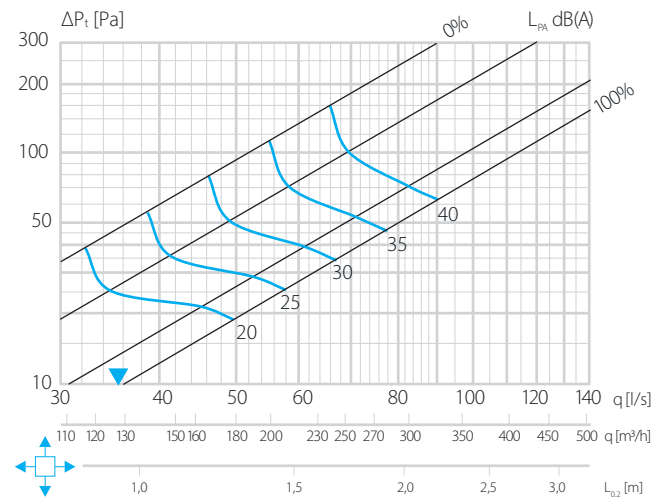
Diagram 01 - PLI-160 - TK-160-160 sound
