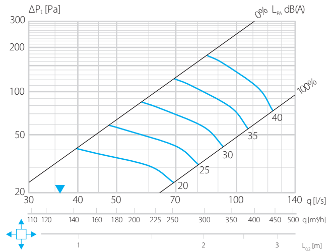
Diagram 07 - PLI-200 - TK-200-160 sound
