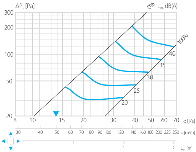
Diagram 04 - PLI-160 - TK-160-100 sound
