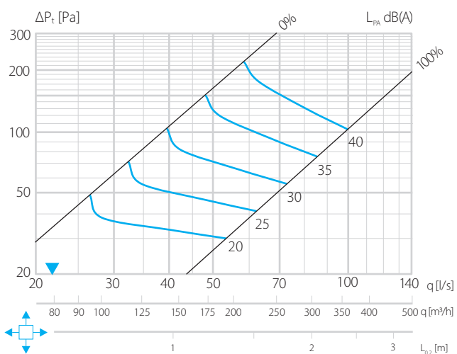
Diagram 06 - PLI-200 - TK-200-125 sound
