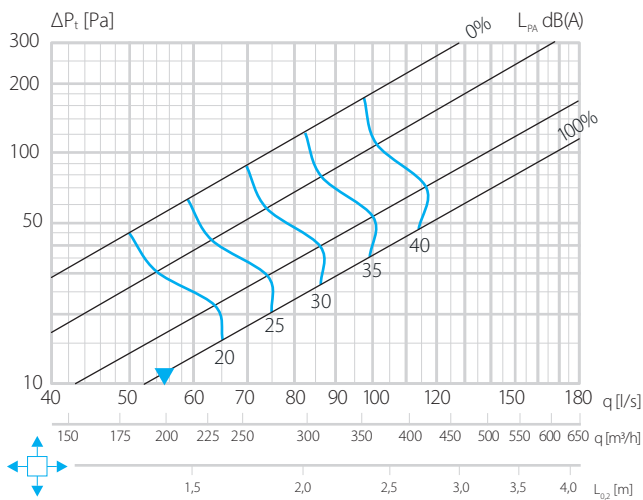
Diagram 02 - PLI-200 - TK-200-200 sound
