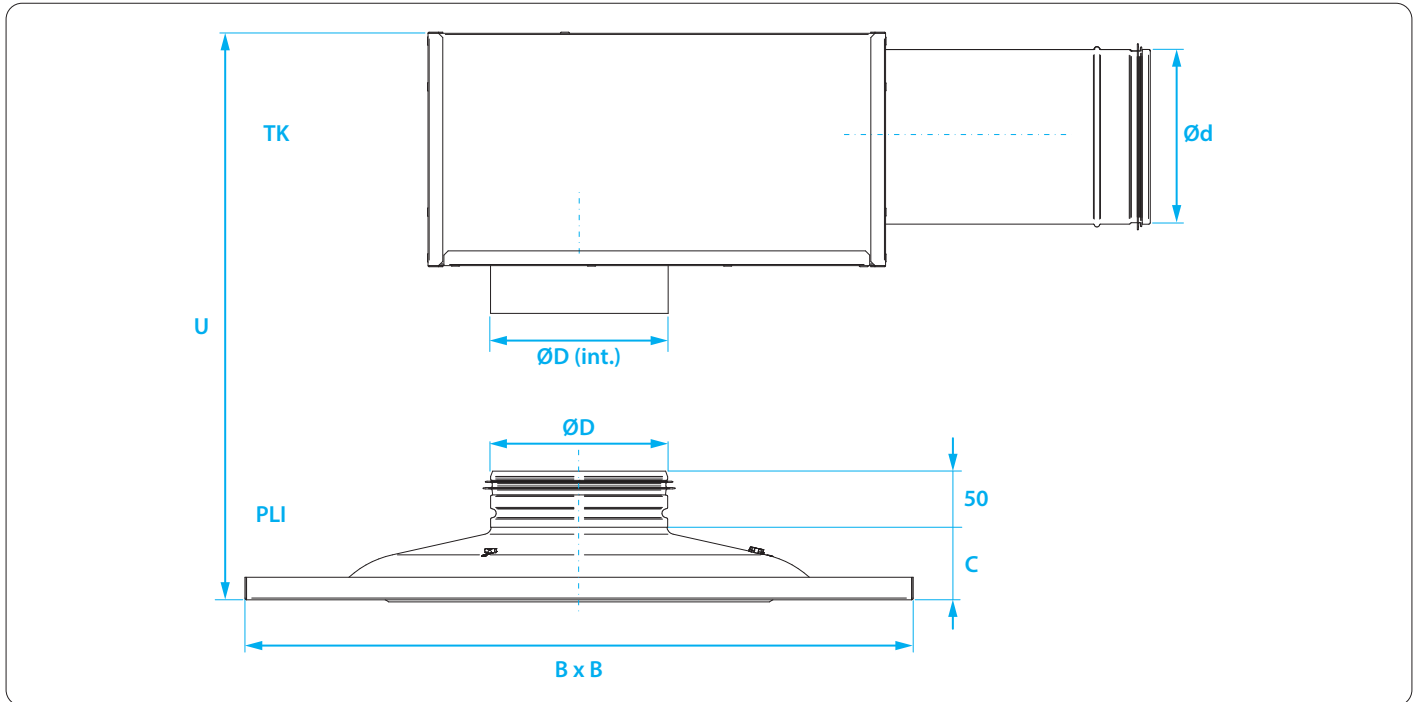
Figure 05 - Dimensions PLI + TK 0-step
